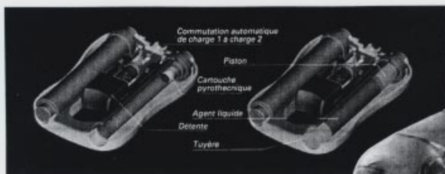
Eclaté du Guardian Angel.
